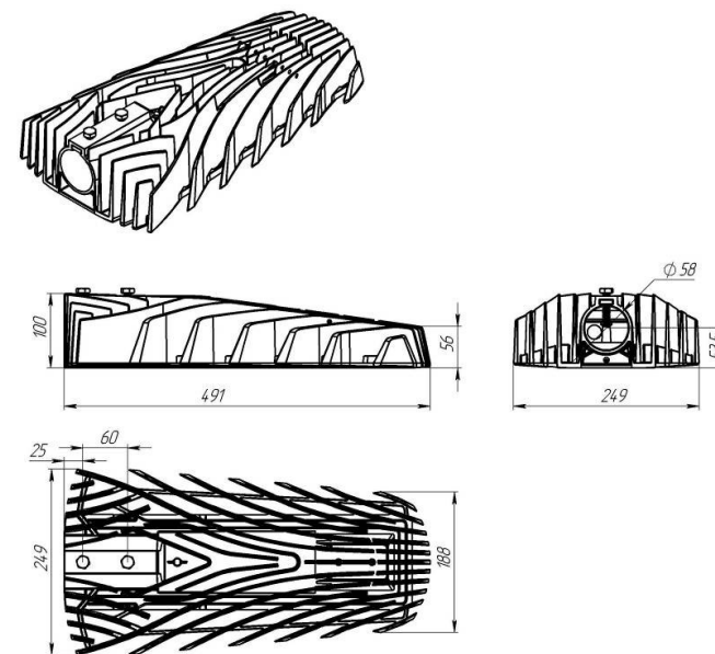
Рисунок 1 Габаритные размеры светильника « Superstreet»
